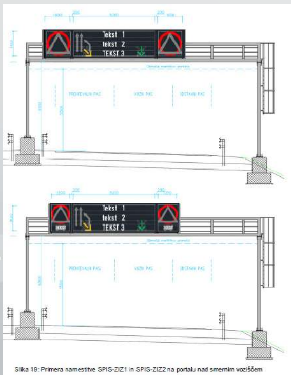
Slika 19: Primera namestitve SPIS-ZIZ1 in SPIS-ZIZ2 na portalu nad smernim voziščem
